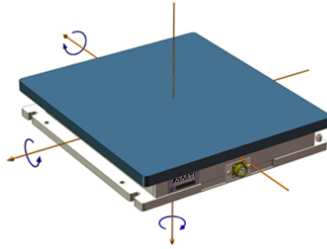
Figura 1. Plataforma de Fuerza Por AMTI, https://www.amti.biz/images/0R6-7-forces-diagram.jpg
