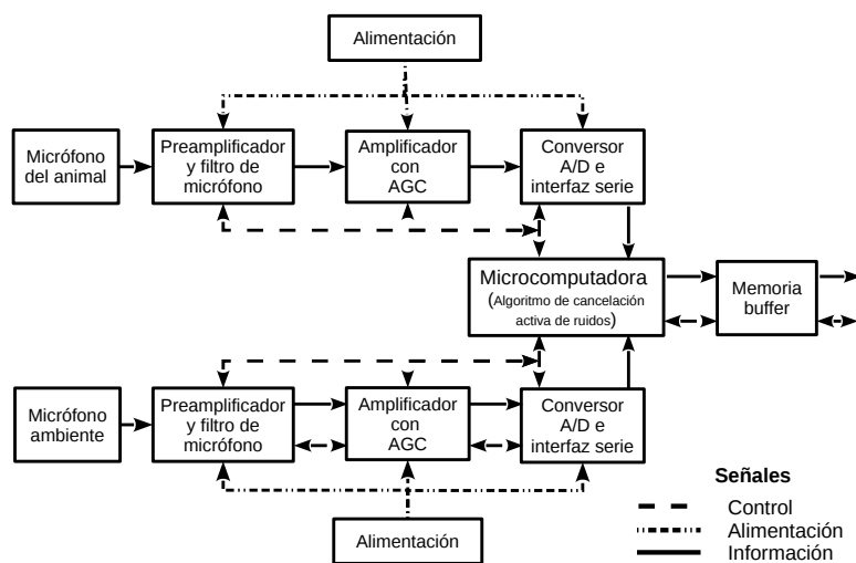
Figura 3: Diagrama de bloques del módulo de adquisición.
