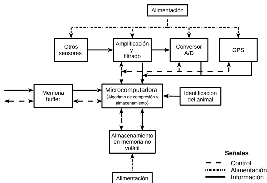
Figura 4: Diagrama del módulo de compresión y almacenamiento.
