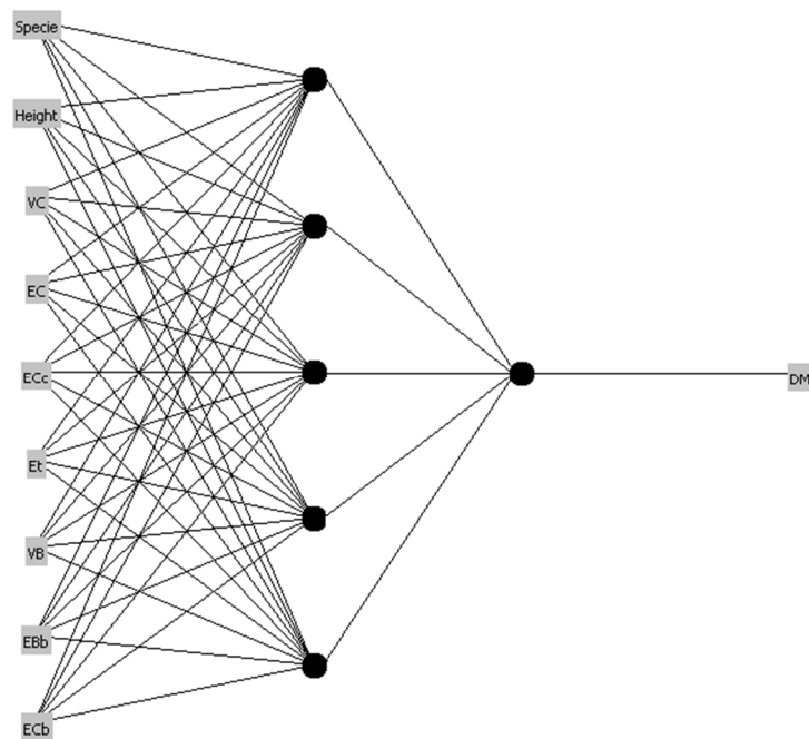
Fig. 2. Esquema del perceptrón con las 10 entradas en la capa de entrada, 5 neuronas en la capa oculta y la salida, en nuestro caso el DMI.
